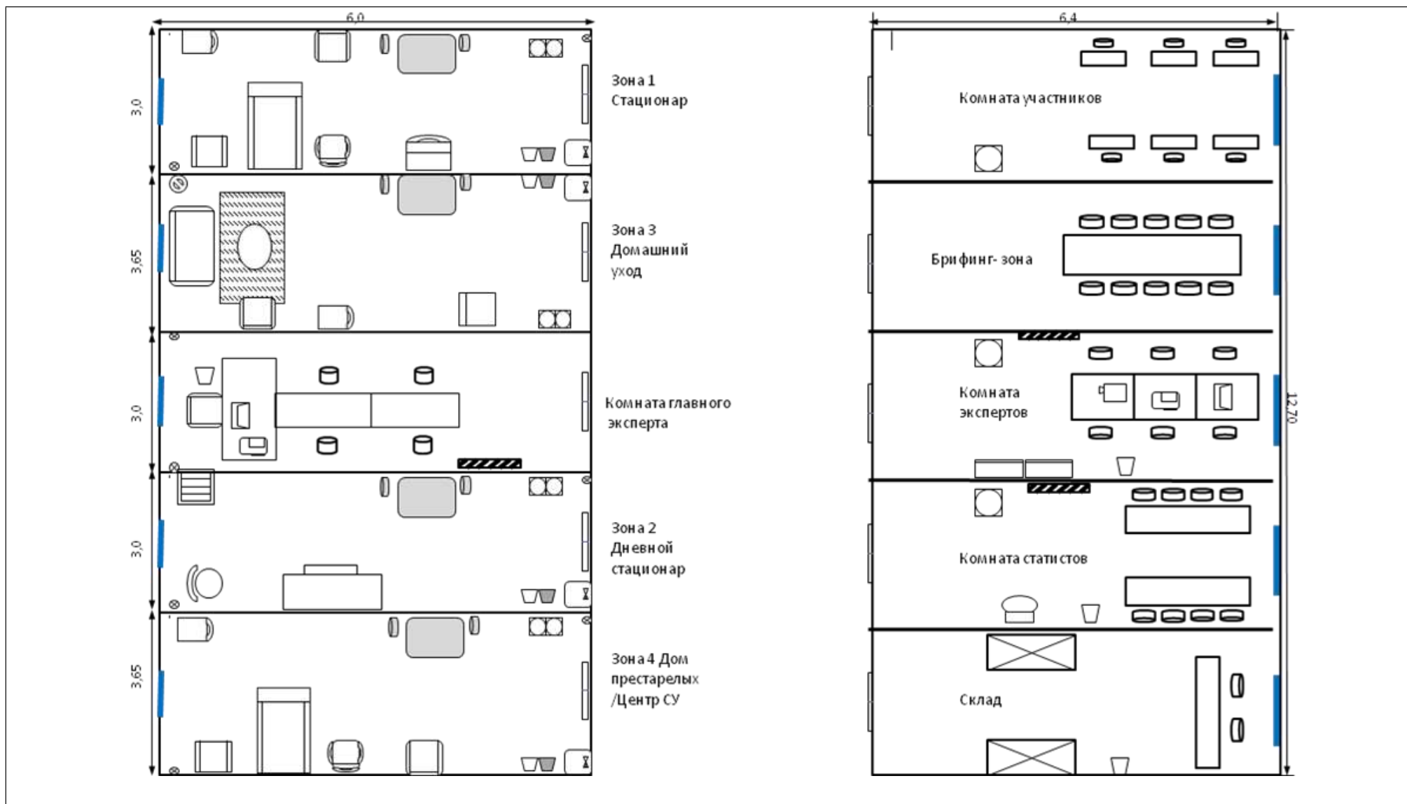
Компоновка оргтехники, спец. приборами согласно ИЛ
